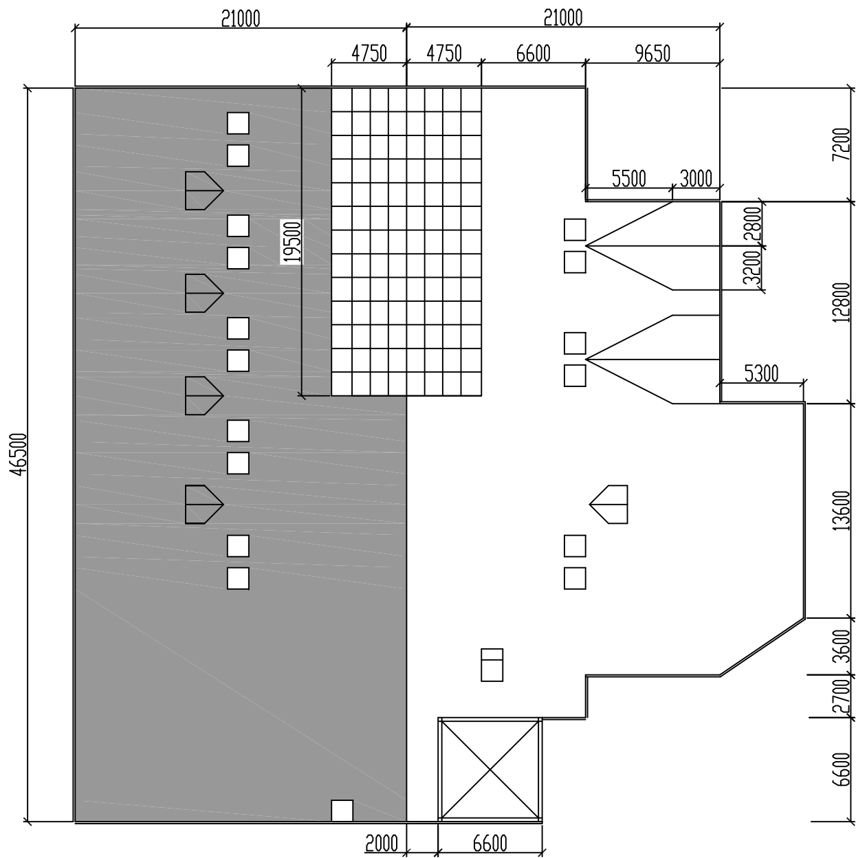
滨湖食堂屋面展开图
