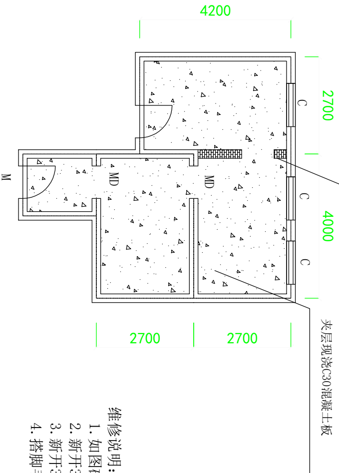
2楼夹层平面图
