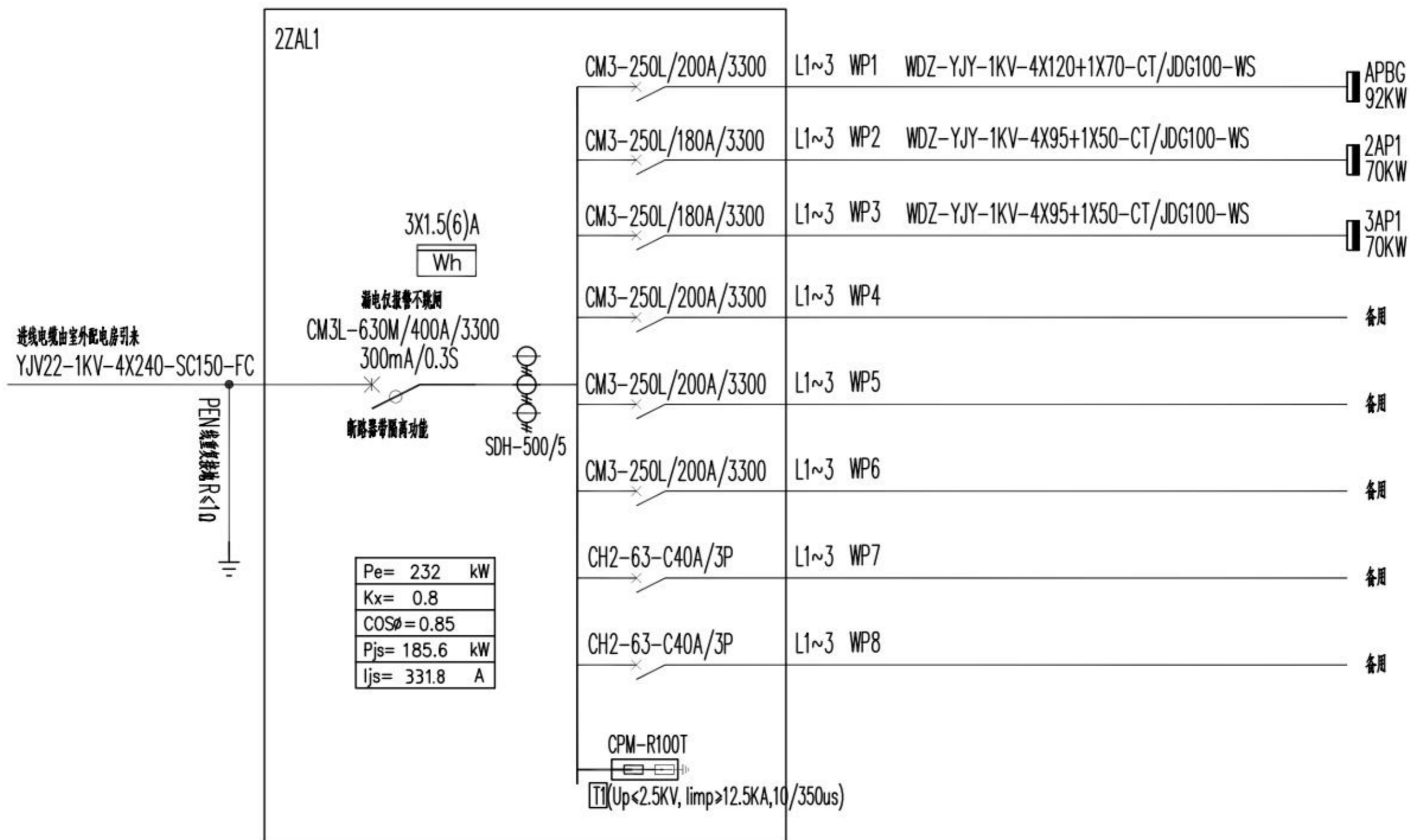
楼栋配电总箱2ZAL1
